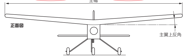
図 7-2 ラジコン飛行機の各部の寸法などを表すための名称。
